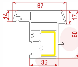
Moving Mullion Profile Hareketli Ortakayıt Profili
