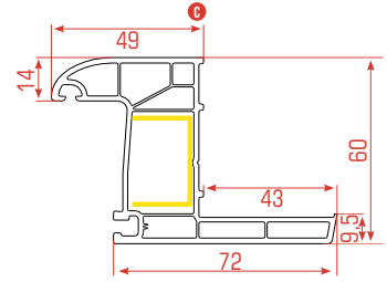
Renovation Frame Profile Pervazlı Kasa Profili بروفيل الإطار مع حاجب
