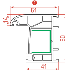
Frame Profile Kasa Profili بروفيل الإطار
