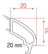
Double Glazing Bead Profile Çift Cam Çita Profili بروفيل نافذة للزجاج المزدوج
