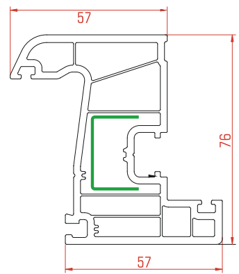
Sash Profile Kanat Profili بروفيل الجناح
