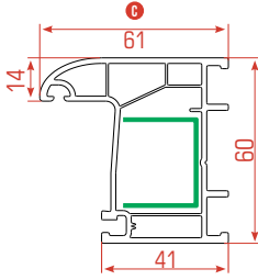
Frame Profile Kasa Profili بروفيل الإطار
