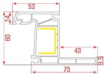
Renovation Frame Profile Pervazlı Kasa Profili بروفيل الإطار مع حاجب
