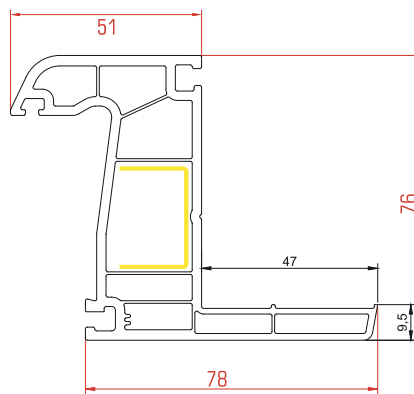
Renovation Frame Profile Pervazlı Kasa Profili بروفيل الإطار مع حاجب
