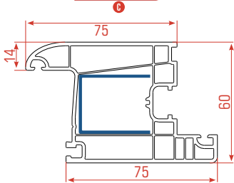
Narrow Inside Opening Door Sash Profile Dar İçe Açılır Kapı Kanat Profili بروفيل جناح باب ضيق يفتح للداخل
