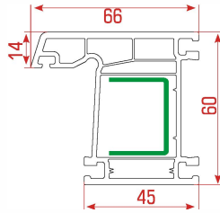
Super Frame Profile Super Kasa Profili بروفيل الإطار الفائق
