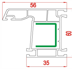
Frame Profile Kasa Profili بروفيل الإطار
