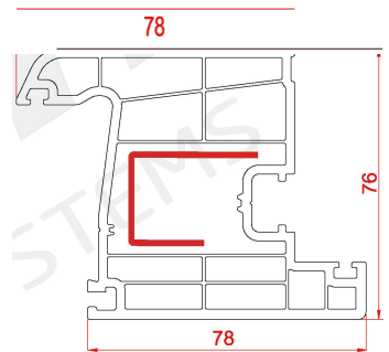
Door Sash Profile
