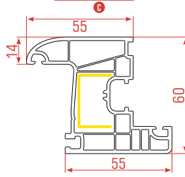
Sash Profile Kanat Profili بروفيل الجناح
