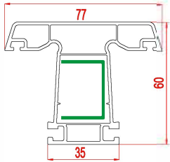
Mullion Profile Ortakayıt Profili
