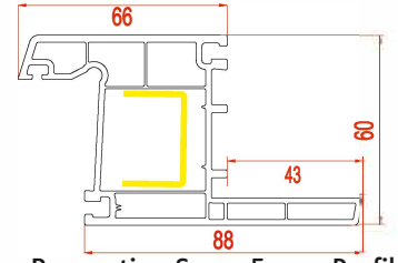
Renovation Super Frame Profile Pervazlı Super Kasa Profili بروفيل إطار فائق للتجديد مع الحلية
