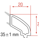
Double Glazing Bead Profile Çift Cam Çita Profili بروفيل نافذة للزجاج المزدوج
