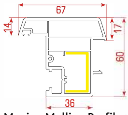
Moving Mullion Profile Hareketli Ortakayıt Profili بروفيل متوسط متحرك "تقابل الجناحين"
