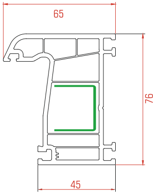
Frame Profile Kasa Profili بروفيل الإطار
