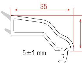
Single Glazing Bead Profile Tek Cam Çita Profili بروفيل نافذة أحادية الزجاج
