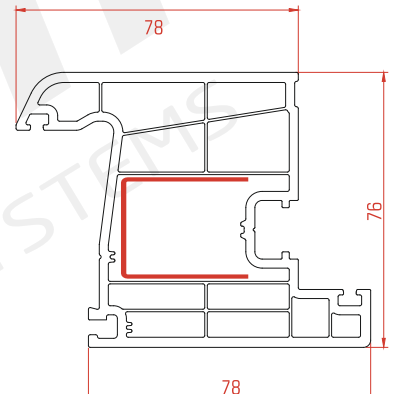
Door Sash Profile Kapi Kanat Profili بروفيل جناح باب
