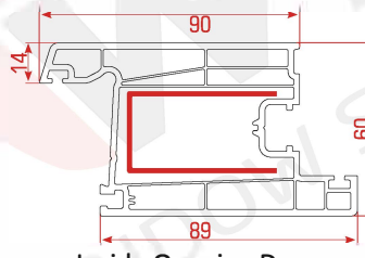
Inside Opening Door Sash Profile İçe Açılır Kapı Kanat Profili بروفيل باب يفتح باتجاه الداخل
