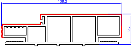
İç Kapı Profili Interior Door Profile بروفيل باب داخلي
