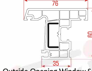
Outside Opening Window Sash Profile Dış Açılır Pencere Kanat Profili بروفيل جناح نافذة يفتح للخارج
