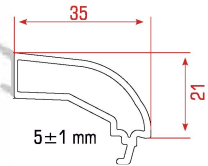
Single Glazing Bead Profile Tek Cam Çıta Profili بروفيل نافذة أحادية الزجاج
