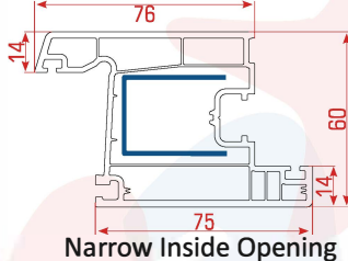
Narrow Inside Opening Door Sash Profile Dar İçe Açılır Kapı Kanat Profili بروفيل جناح باب ضيق يفتح للداخل
