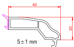
Single Glazing Bead Profile Tek Cam Çita Profili بروفيل نافذة أحادية الزجاج
