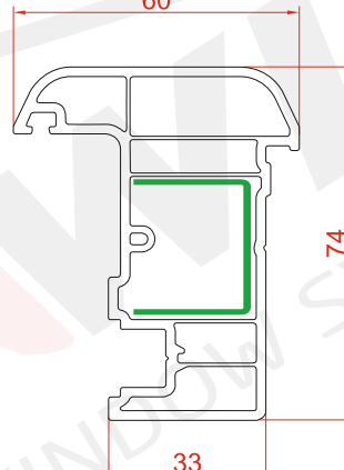
Moving Mullion Profile Hareketli Orta Kayıt Profili بروفيل العمود الوسيط المتحرك
