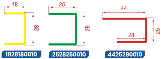
Moving Mullion Profile Hareketli Orta Kayıt Profili بروفيل العمود الوسيط المتحرك
