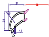
Double Glazing Bead Profile Çift Cam Çita Profili بروفيل نافذة للزجاج المزدوج
