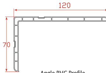
Angle PVC Profile بروفيل بي في سي زاوية
