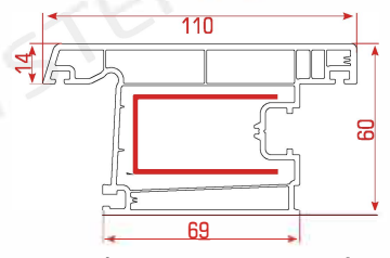
Outside Opening Door Sash Profile Dış Açılır Kapı Kanat Profili بروفيل باب يفتح باتجاه الخارج
