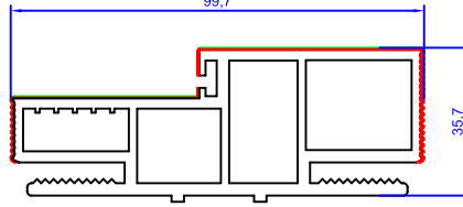
İç Kapı Profili Interior Door Profile بروفيل باب داخلي
