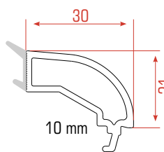
Single Glazing Bead Profile Tek Cam Çita Profili بروفيل نافذة أحادية الزجاج
