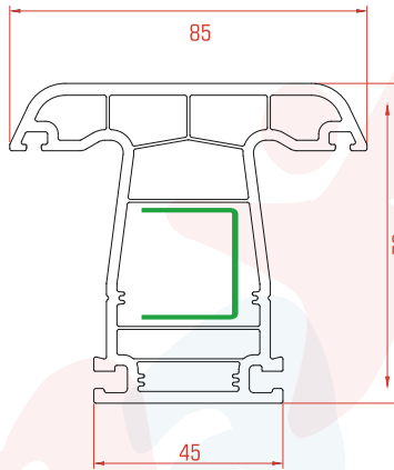
Mullion Profile Ortakavit Profili بروفيل جناح متوسط على شكل T
