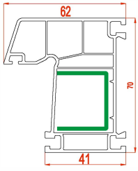
Frame Profile Kasa Profili بروفيل الإطار
