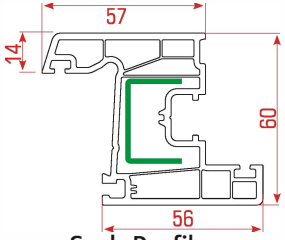
Sash Profile Kanat Profili بروفيل الجناح
