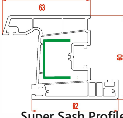
Super Sash Profile Super Kanat Profili بروفيل الجناح الفائق
