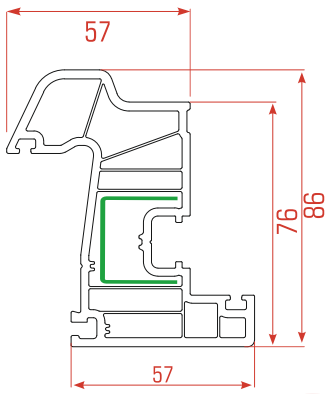
Drainaged Sash Profile Damalıklı Kanat Profili بروفيل جناح مع مصرف المياه
