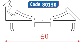
Angled Post Adapter Profile بروفيل محول عمود مائل
