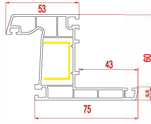
Renovation Frame Profile Pervazlı Kasa Profili بروفيل الإطار مع حاجب
