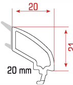
Double Glazing Bead Profile Çift Cam Çıta Profili بروفيل نافذة للزجاج المزدوج
