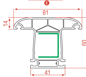
Mullion Profile Ortakayıt Profili بروفيل جناح متوسط على شكل T
