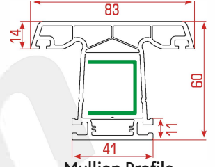
Mullion Profile Ortakayıt Profili بروفيل جناح متوسط على شكل T
