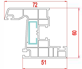
Sash Profile Kanat Profili بروفيل الجناح
