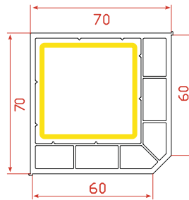
Rectangle Profile Kutu Profili بروفيل مستطيل
